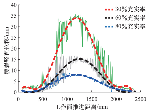
图 6 不同充实率顶板变形曲线
