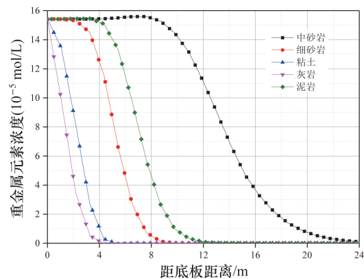
图 14 重金属元素在底板中浓度分布规律
