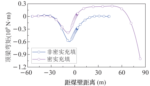
图11 距煤壁不同位置顶梁弯矩趋势
