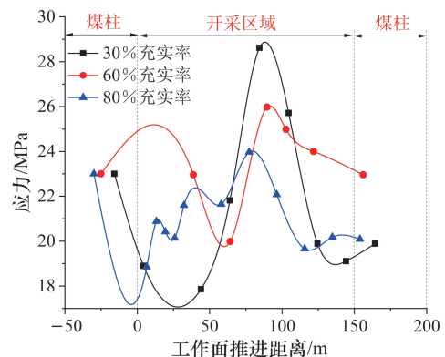
图 7 不同充实率应力变化曲线
