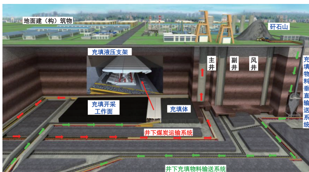
图 1 充填开采技术示意
