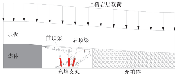
图8 深部充填体、充填支架与围岩相互关系
