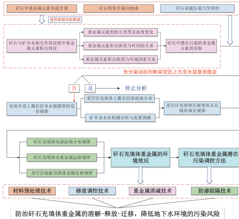
图 15 重金属潜在污染调控设计流程
