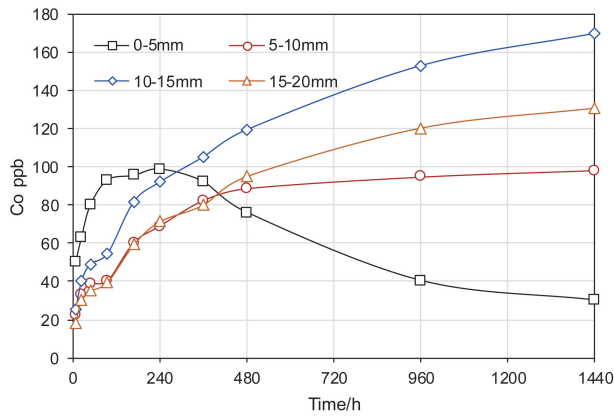
图 13 重金属析出浓度随时间变化曲线
