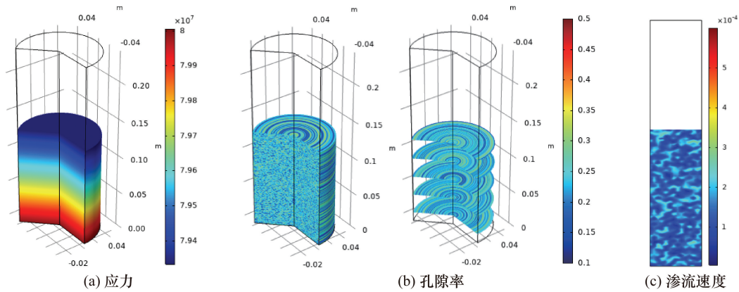
图 4 散体充填物料承载压缩渗流规律
