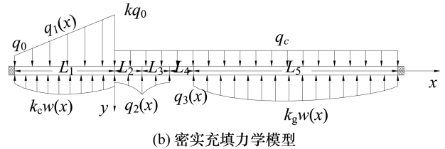
图9 不同充填状态采场顶板力学模型
