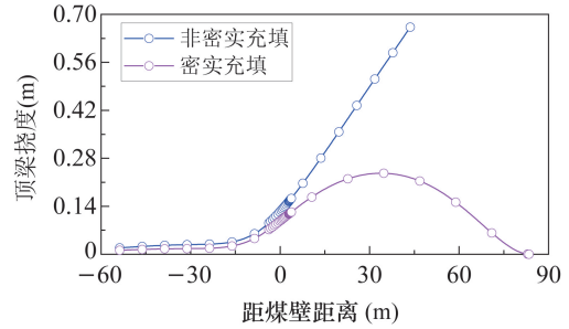
图10 距煤壁不同位置顶梁挠度趋势
