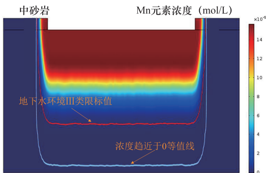
图 14 重金属元素在底板中浓度分布规律
