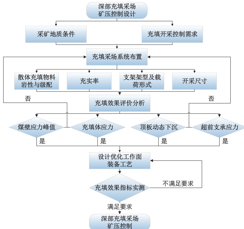
图12 深部充填采场矿压控制方法设计流程
